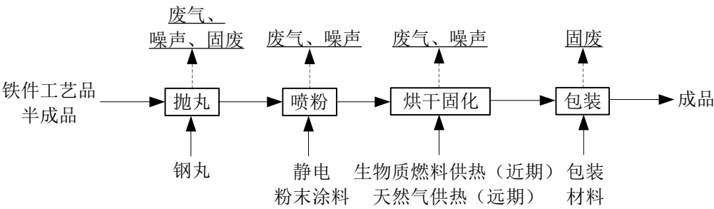
图 4-1 改建前铁件工艺品生产工艺流程图
