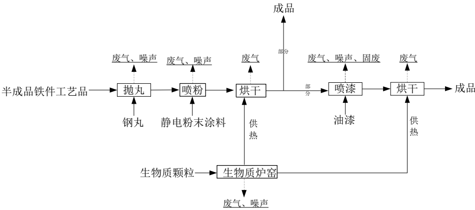
图 4-2 改建后铁件工艺品生产工艺流程图
