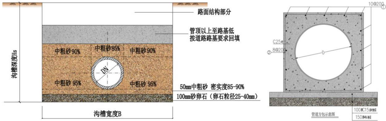
图 4.5-4 典型沿路及沿河污水主管埋设断面示意图
