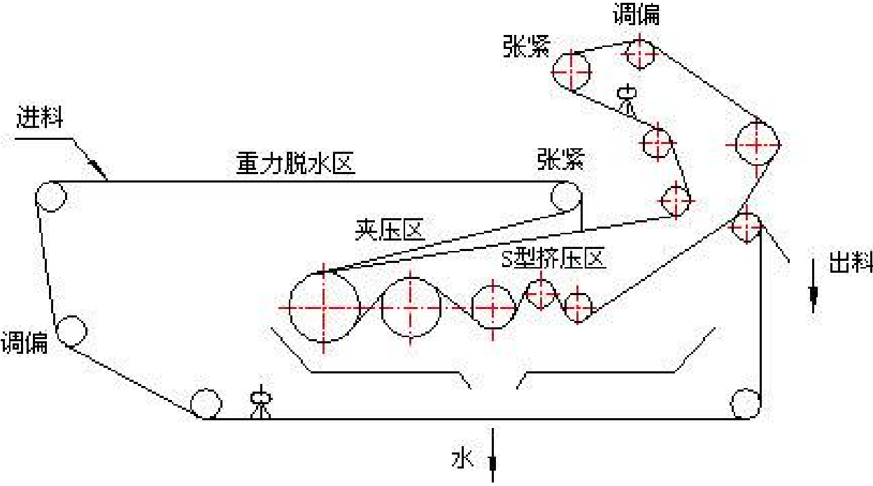
图 4.4-2 带式污泥脱水机原理图
