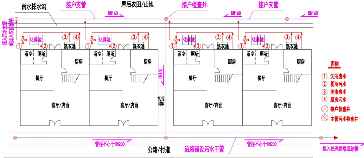
图 4.5-2 典型农村多户联排房屋接户管布置图
