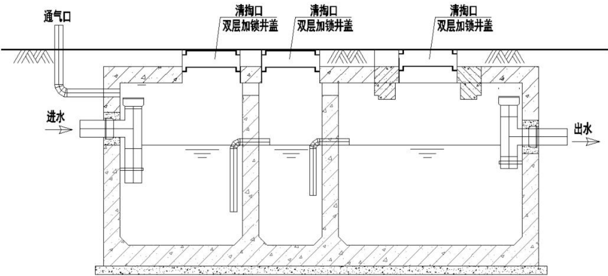
图 4.4-6 户用标准三格化粪池构造示意图
