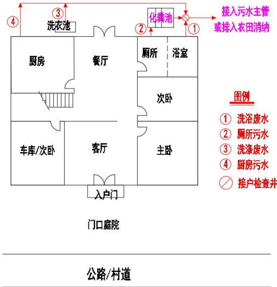
图 4.5-1 典型农村单户房屋接户管布置图
