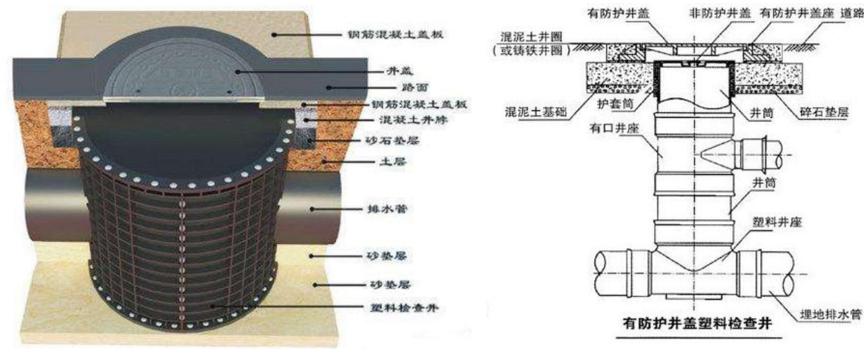
图 4.5-5 典型同材一体化检查井安装示意图
